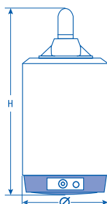
Ventouse position murale
