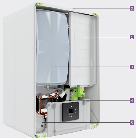
Visuel en coupe du modèle GVT iC 24/42
